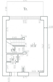
Pirmo aukšto planas
