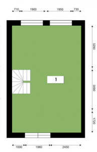
3 aukšto planas
