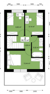
2 aukšto planas
